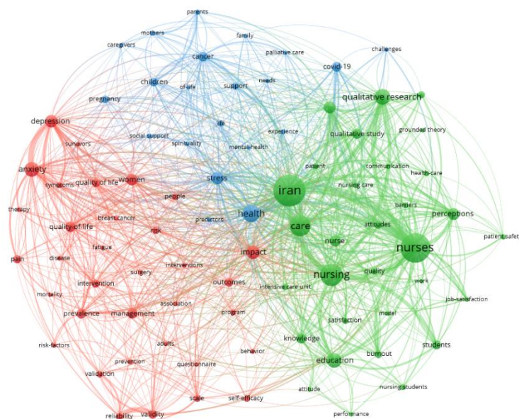
شکل ۵. شبکه هم‌رخدادی کلمات کلیدی نویسنده‌ها
